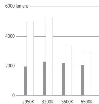
Source Four LED Série 1 Lustr+ vs Source Four LED Série 2 Lustr Des blancs plus intenses
