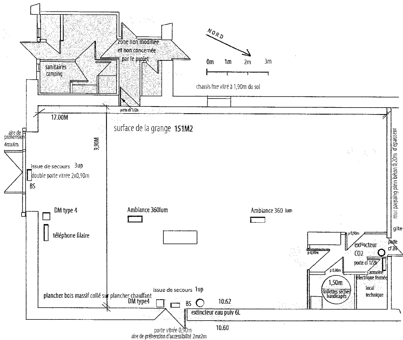
Plan de la grange, projet
