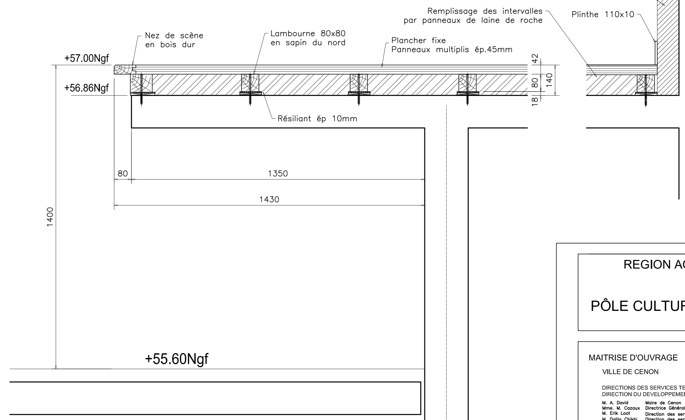
Coupe B-B
