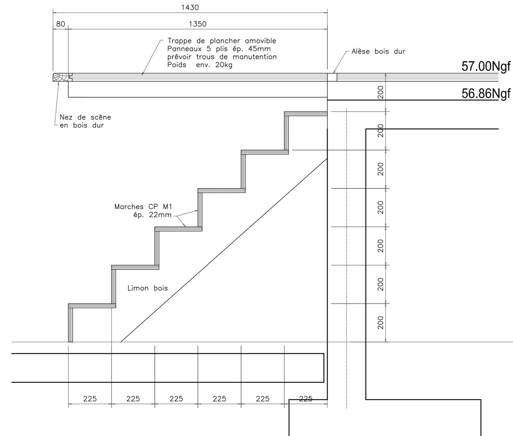
Coupe A-A sur escalier d'accès à la scène
