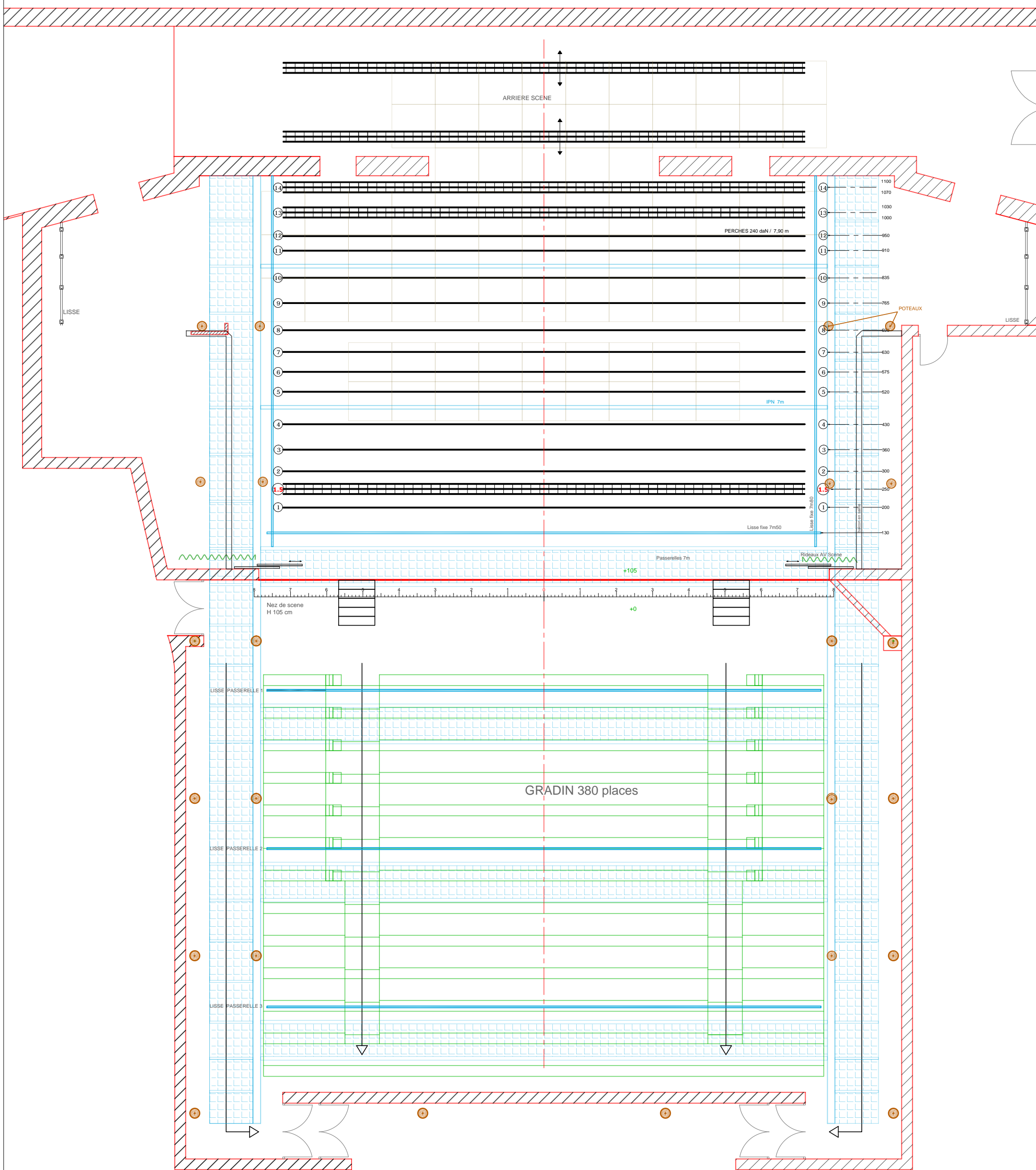
Théâtre de l'Union- Limoges. scène salle1/100
