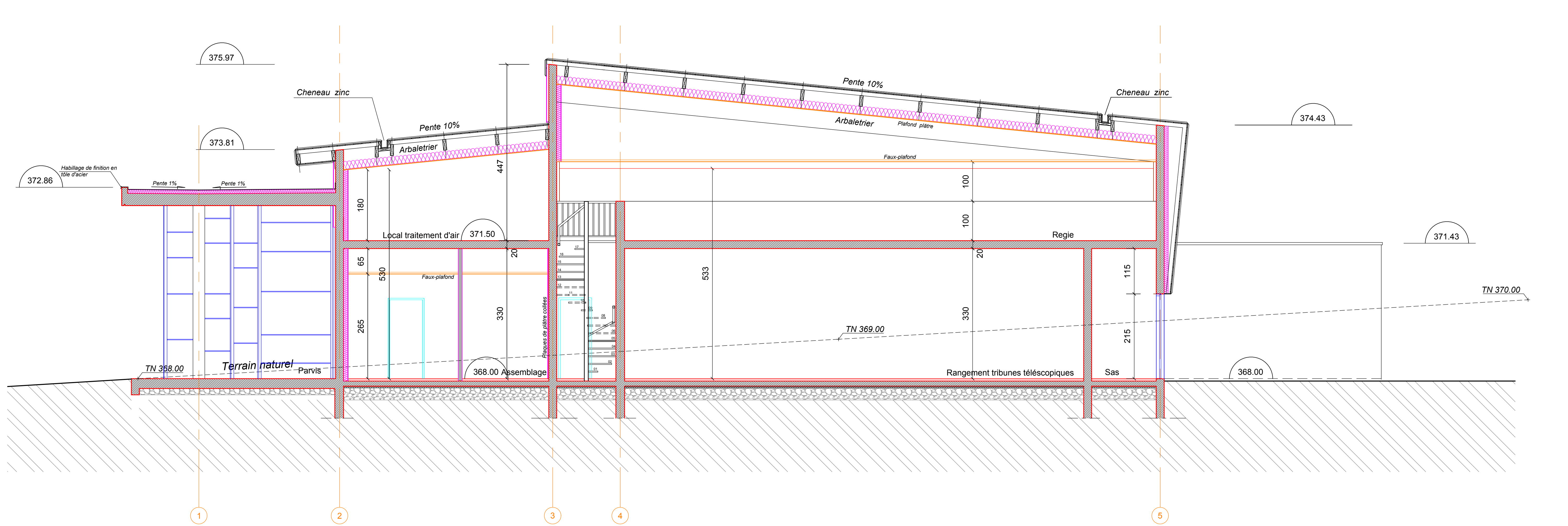
Coupe BB
