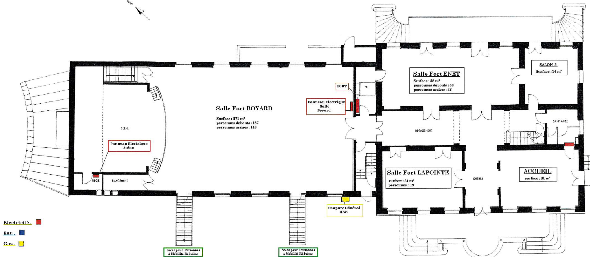
PLAN DU REZ DE CHAUSSEE
