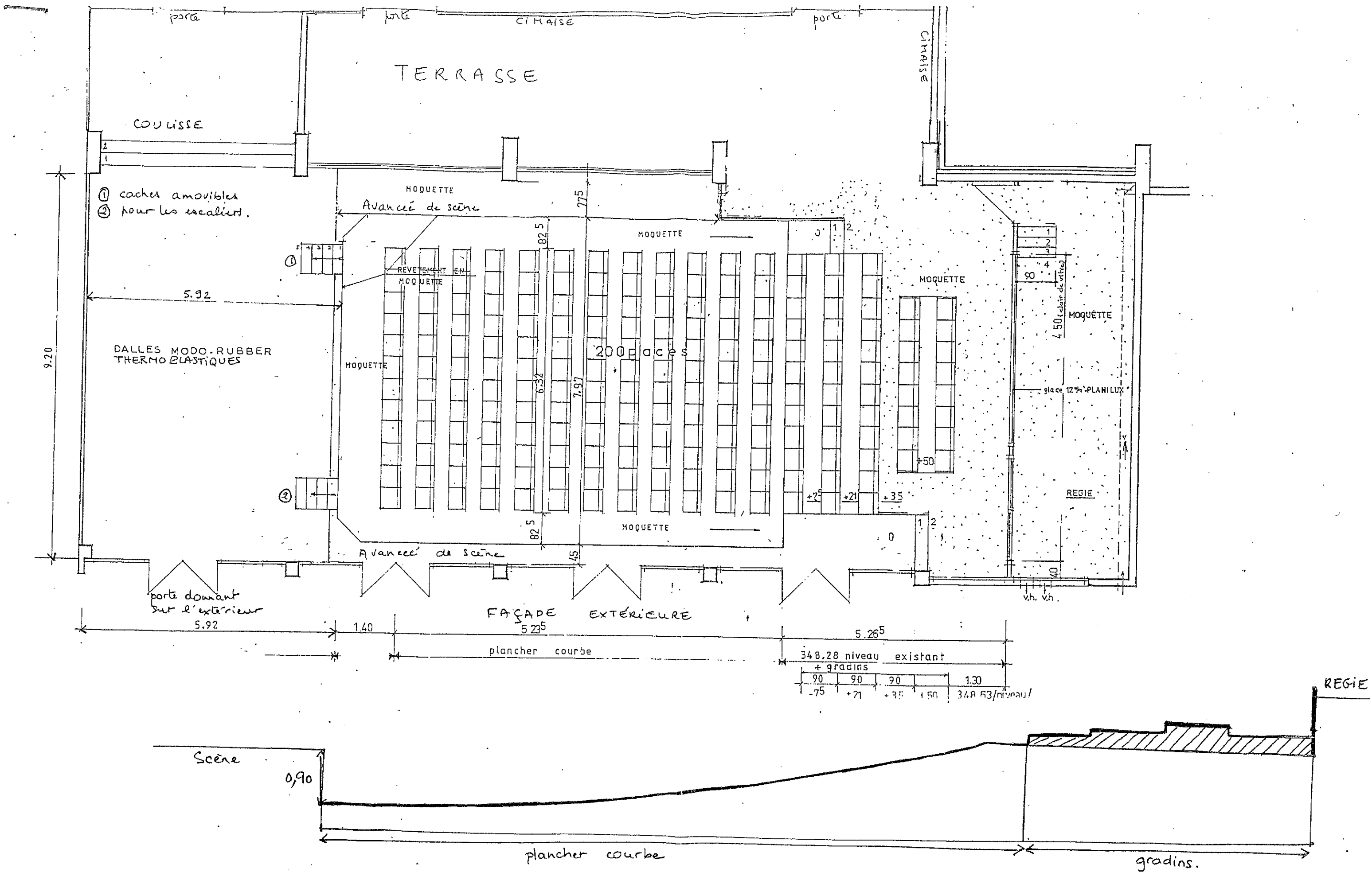
SALLE N°2. BEAUBREUIL. Plan d'ensemble et coupe agrandie
