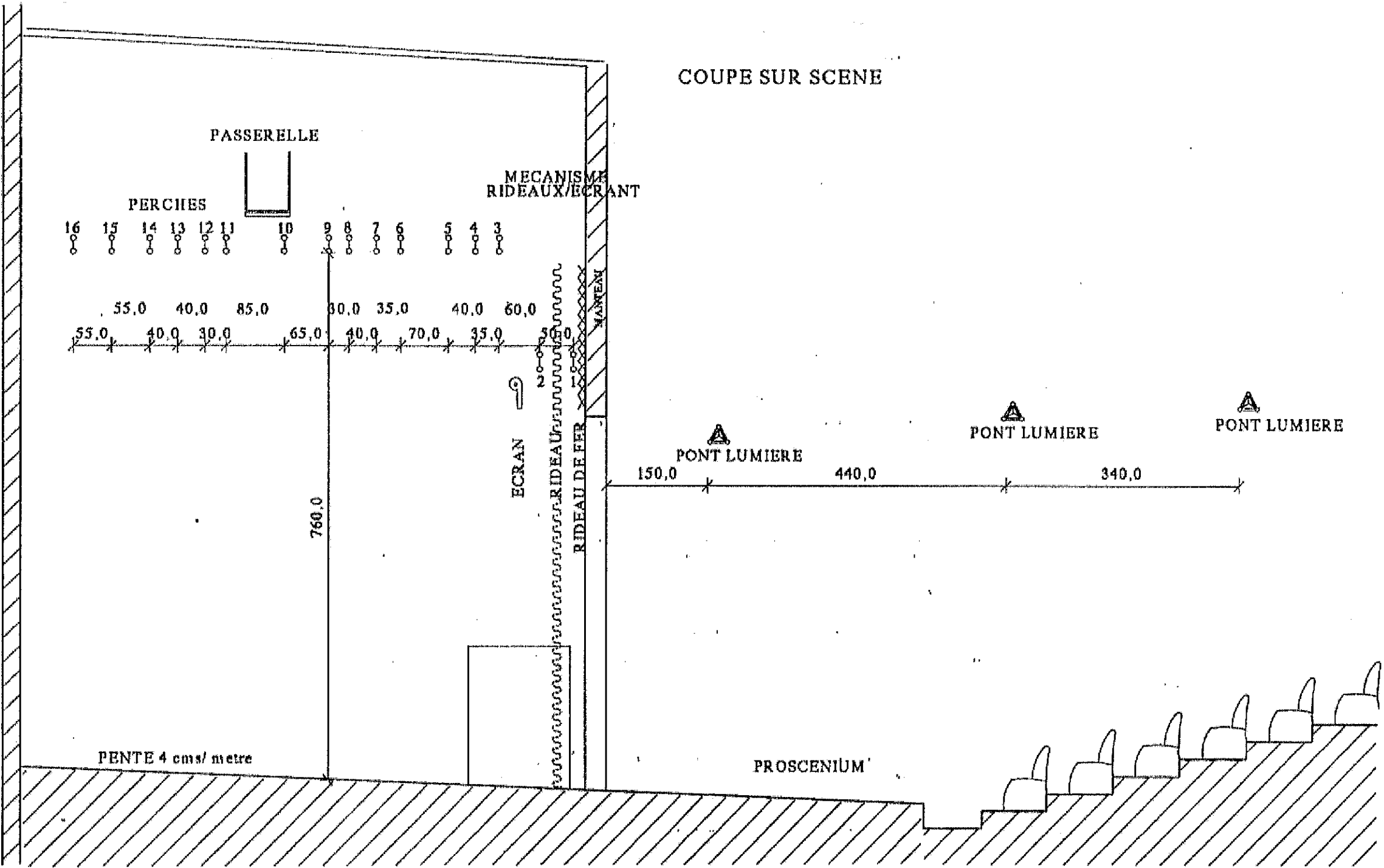
COUPE A-A
