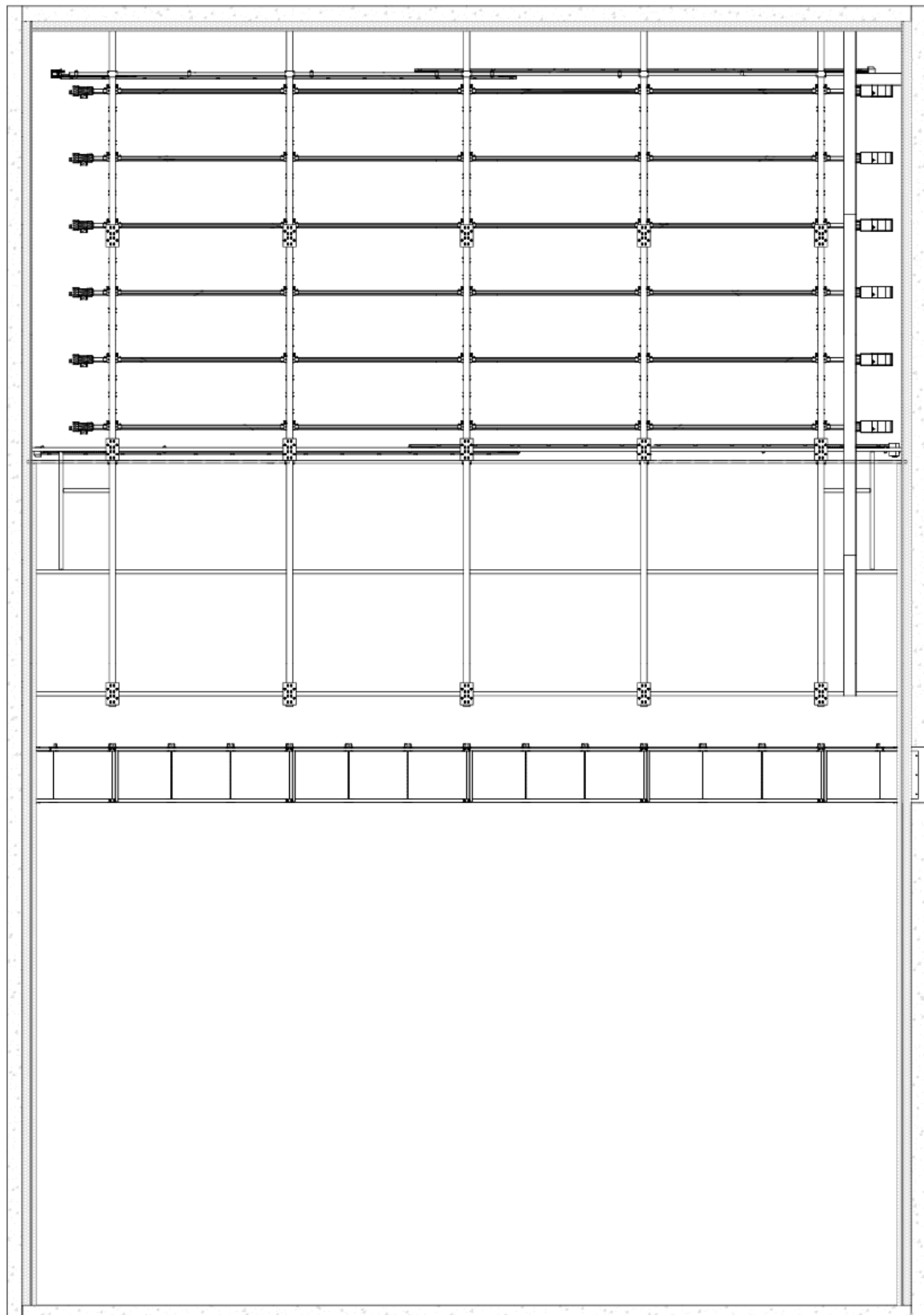
Vue en plan niveau Faux-gril (1:50)
